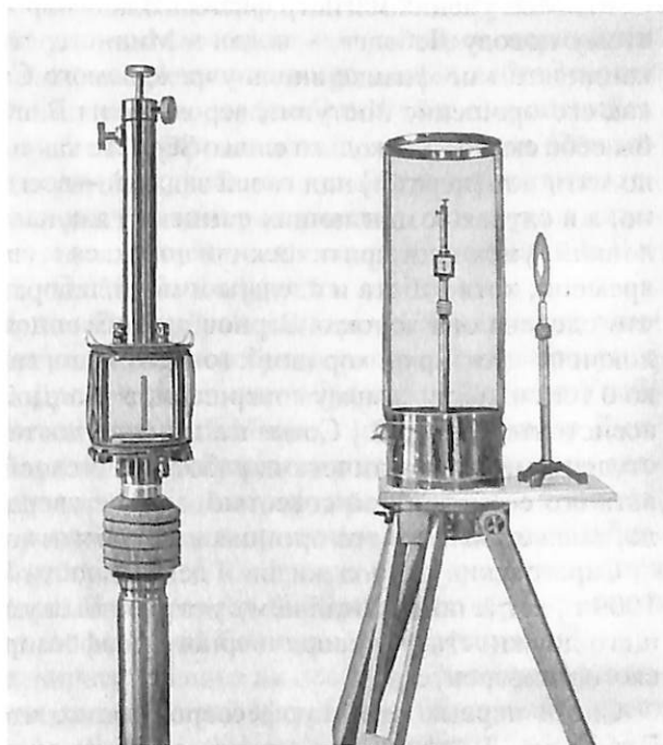
Портативный фометр Лебедева – Зёрнова
