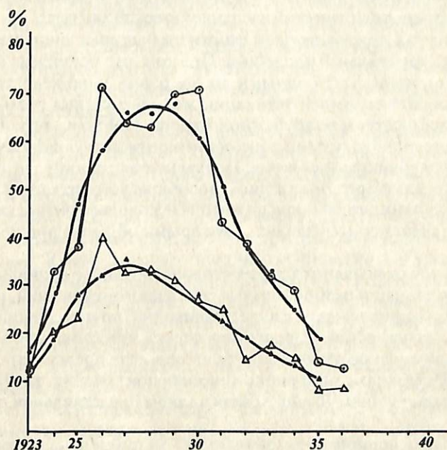
Рис. 4. Вклад советских физиков в «Zeitschrift für Physik» (по книге: Paul Josephson. Physics and Politics in Revolutionary Russia. Berkeley, 1991.) Кружки — число статей на соответствующий год Треугольники — процент статей из СССР от общего числа статей за год в журнале Тонкие линии — конкретные значения на соответствующий год Толстые линии — сглаженные средние
