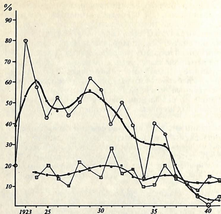
Рис. 1. Доля публикаций на иностранных языках в продукции советских математиков Круги — публикации за границей Квадратики — публикации на иностранных языках в СССР Тонкие линии — конкретные значения на соответствующий год Толстые линии — сглаженные средние
