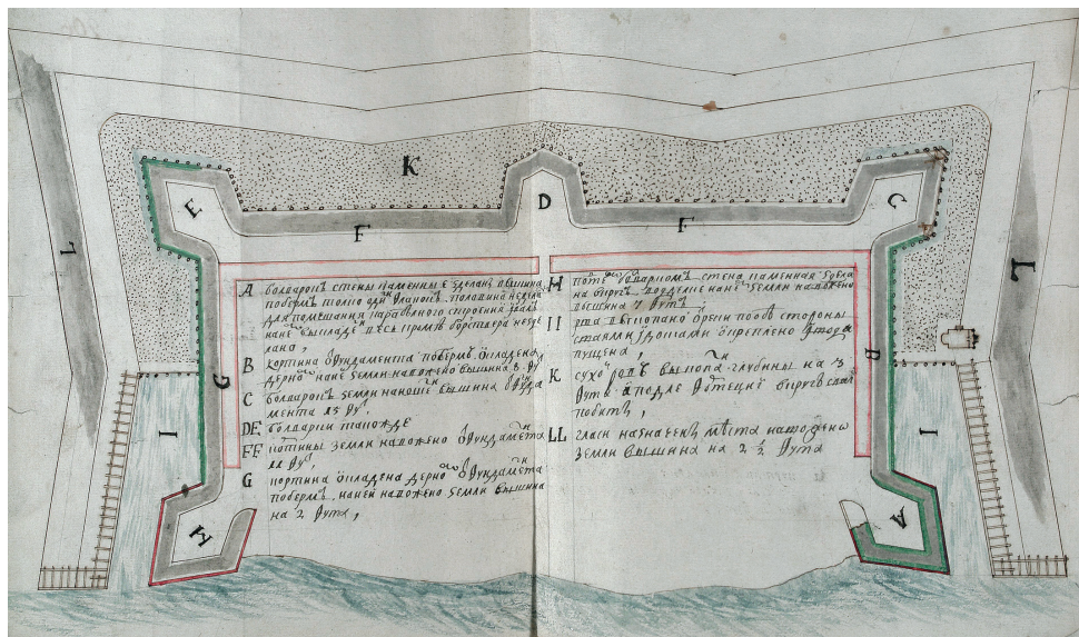
Чертеж Адмиралтейской крепости с указанием проводимых работ по укреплению фортификационных сооружений, 1716 г. Подлинник (РГАДА. Ф. 9. Оп. 3. Отд. 2. Д. 28. Л. 206–206а)
